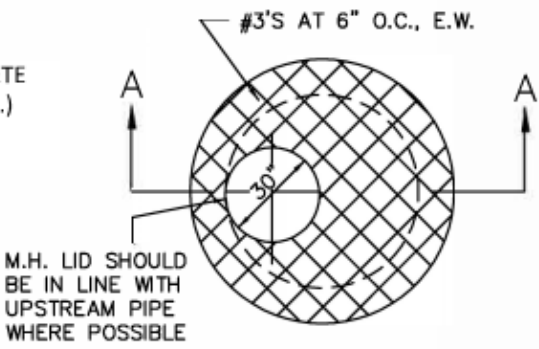
ROOF STEEL LAYOUT N.T.S.
