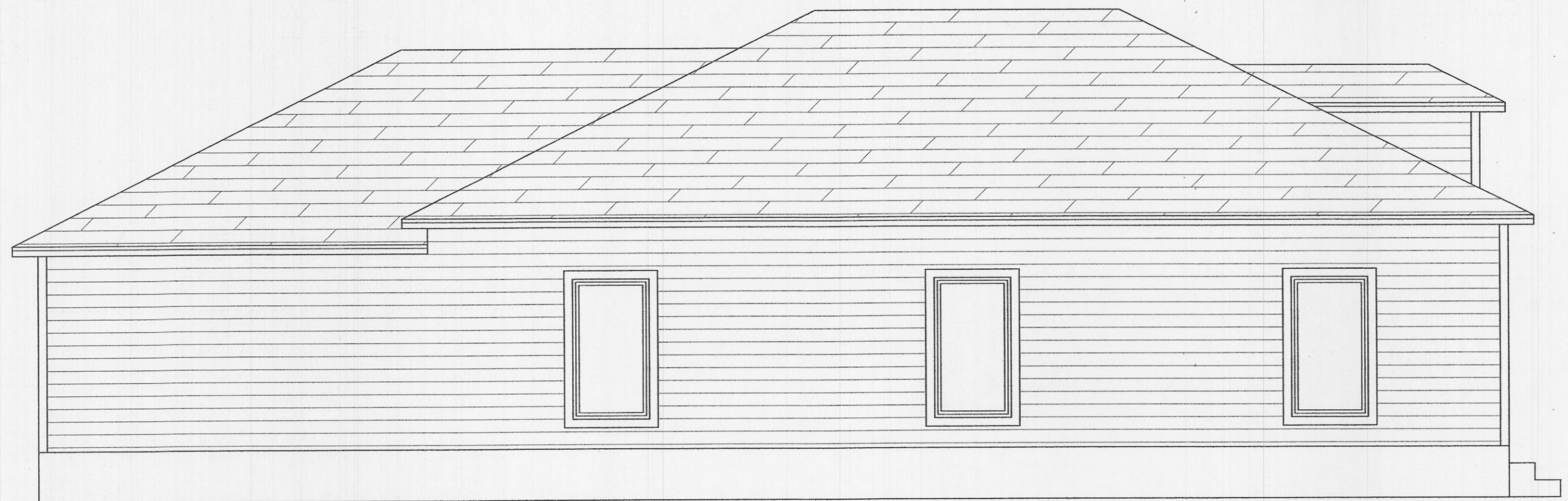
④ LEFT ELEVATION SCALE: 1/4"=1'-0"
